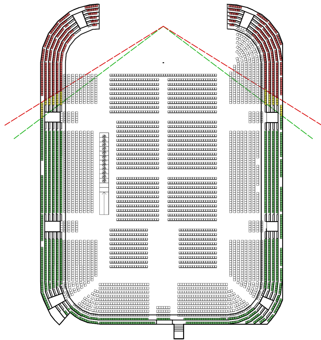
1 | UPPER Scale: 1:500
