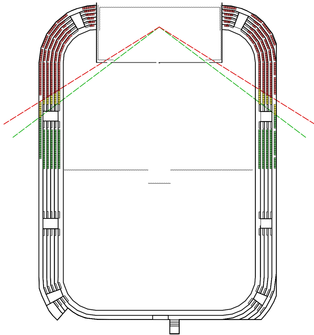
3 | UPPER Scale: 1:500
