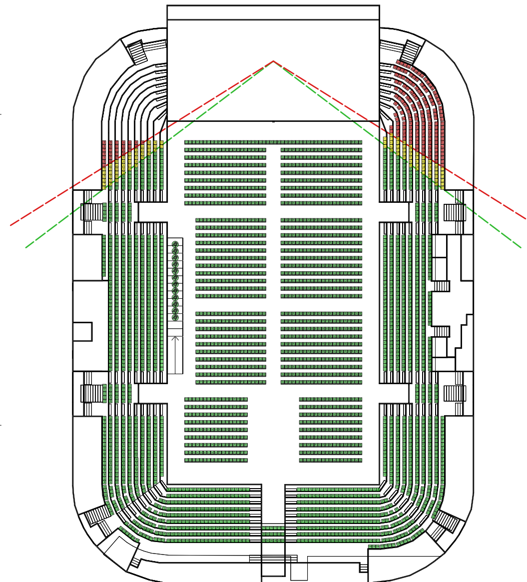
4 | LOWER Scale: 1:500
